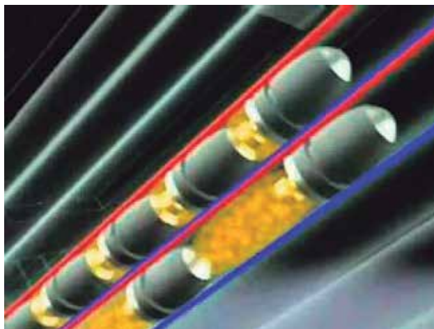
Disposición de los proyectiles en el tubo cañón, en el tubo inferior se aprecia el momento del disparo.
